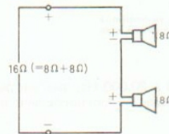
CONNEXION EN SERIE SERIENANSCHLUSS SERIES CONNECTION
