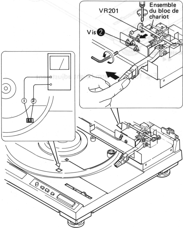
Fig. 13-2 Réglage du gain du sensor d'alignement et du décentrage
