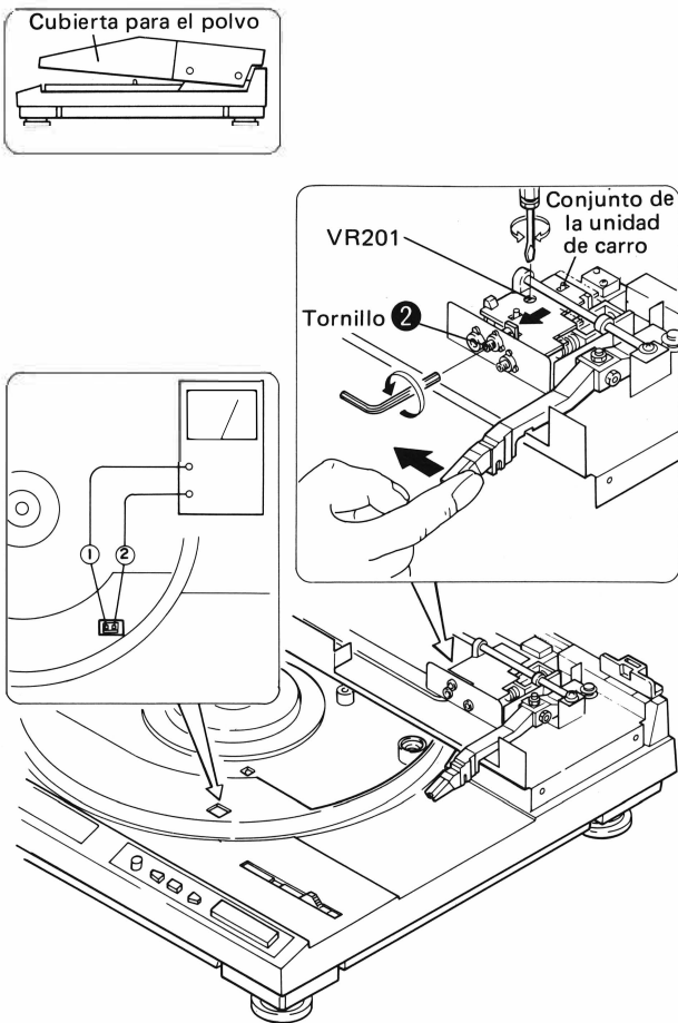
Fig. 13-2 Ganancia del sensor de seguimiento y ajuste de descentrado
