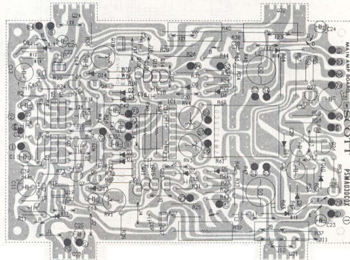
PSMA030COX, AF Power Amplifier
