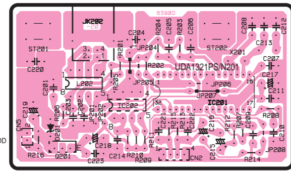
P.C.B. AMP(4)
