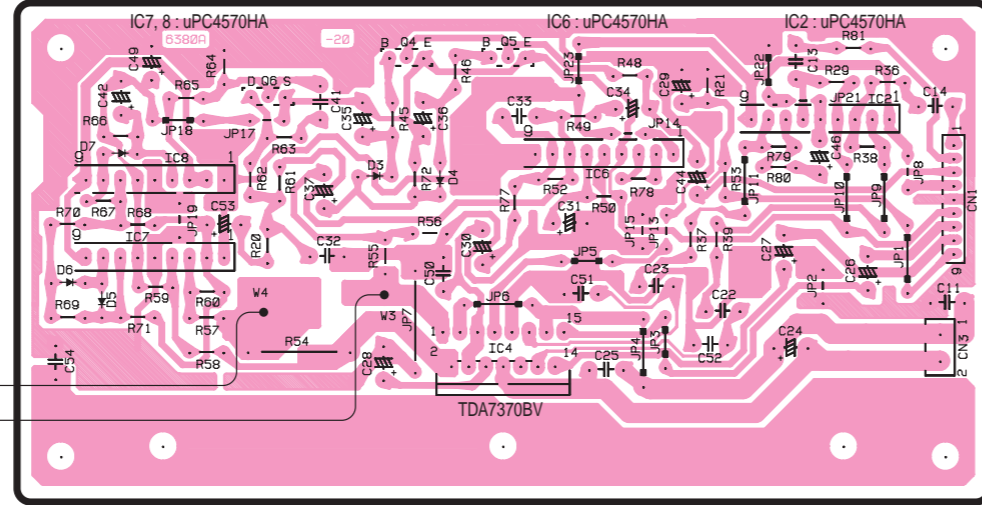
P.C.B. AMP(1)
