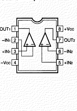
IC2, 805 : KIA4558 Dual OP-Amp
