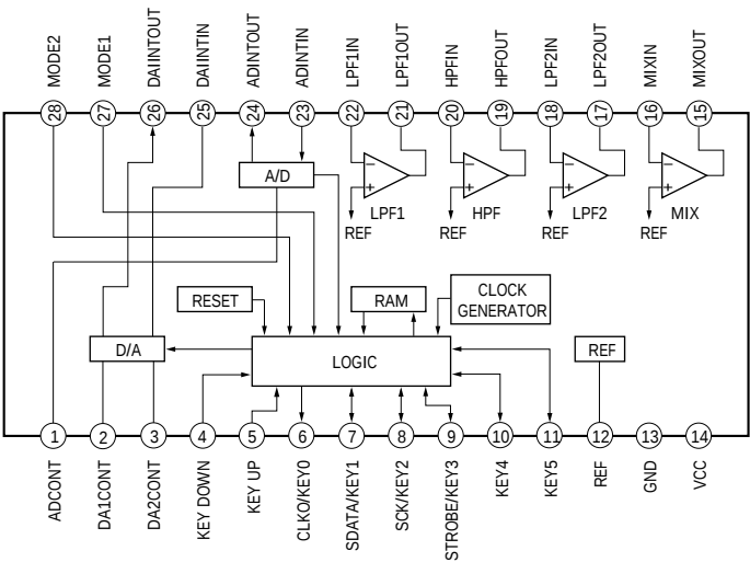
IC6003 M65847FP
