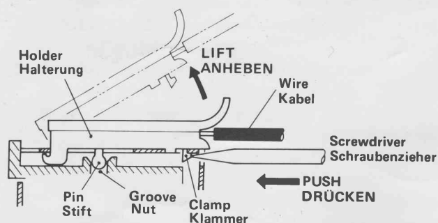
Disconnecting the wire Entfernen des Kabels
