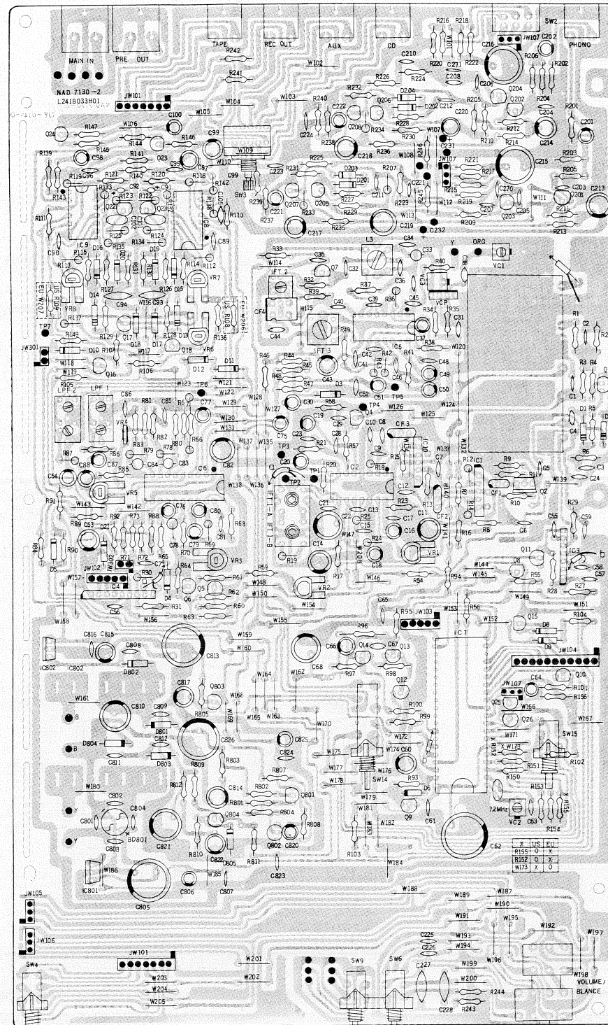
DISPLAY PCB
