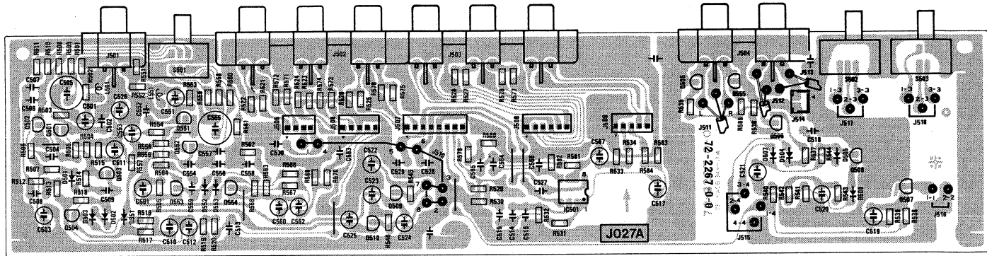
INPUT/OUTPUT P.C.B. ASS'Y (J027A)
