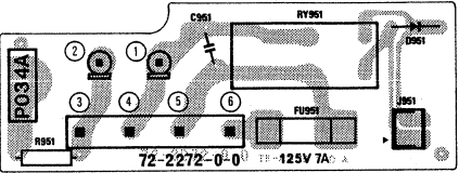
MAINS INPUT P.C.B. ASS'Y (P034A)
