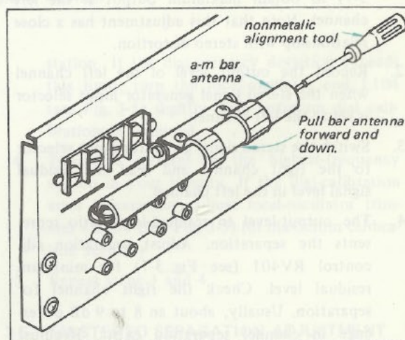
Fig. 3-9. A-m bar antenna core alignment
