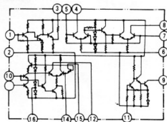
IC202 AN217
