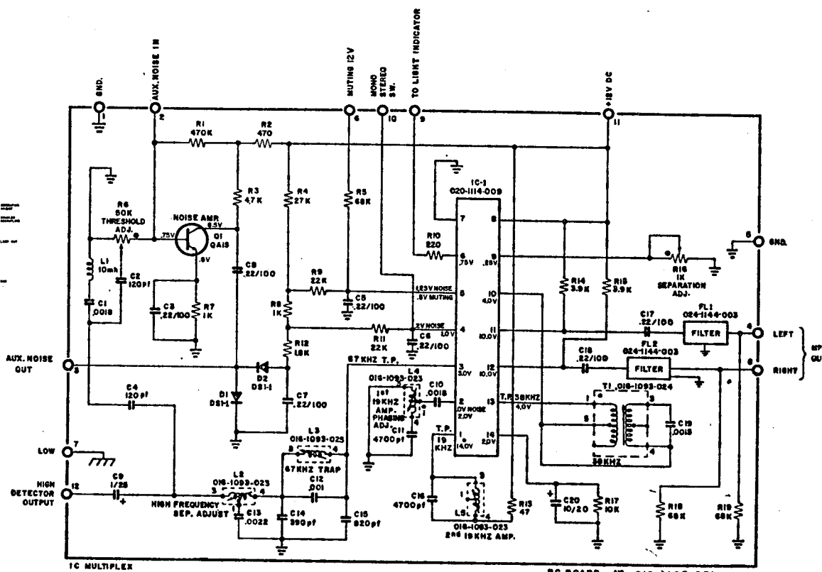
PC BOARD Nº 019-1107-071
