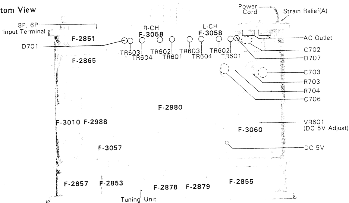
Parts List &lt;Top &amp; Bottom View&gt;
